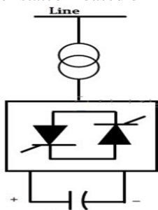
Fig. 6 STATCOM structure
