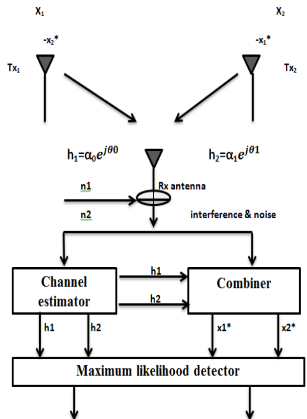
Fig 3. STBC Decoder
