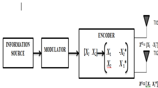
Fig 2. STBC Encoder
