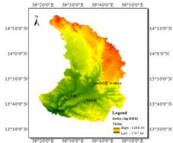
Fig.2. SRTM 30*30 DEM of Geba watershed
