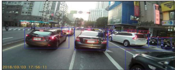
Fig.2. YOLO Detection
