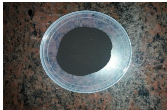
Fig 2.2. lignin
